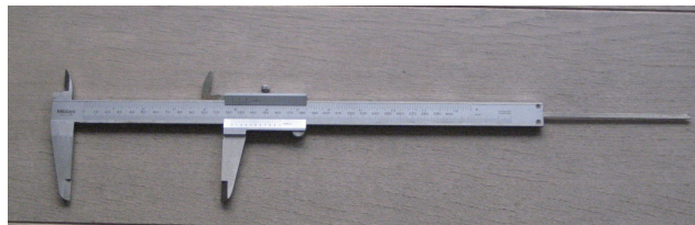
Εικόνα 10: Μεγαλύτερο παχύμετρο
