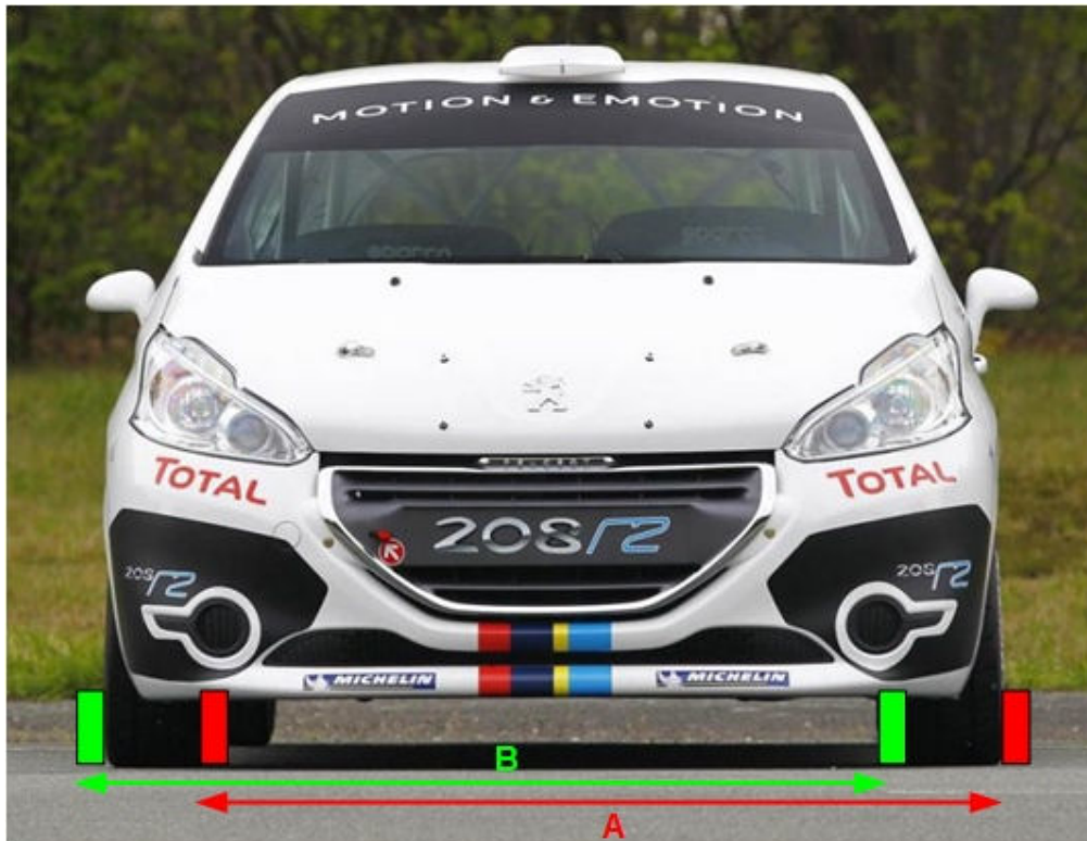
Εικόνα 54: Μέτρηση μετατρόχιου
