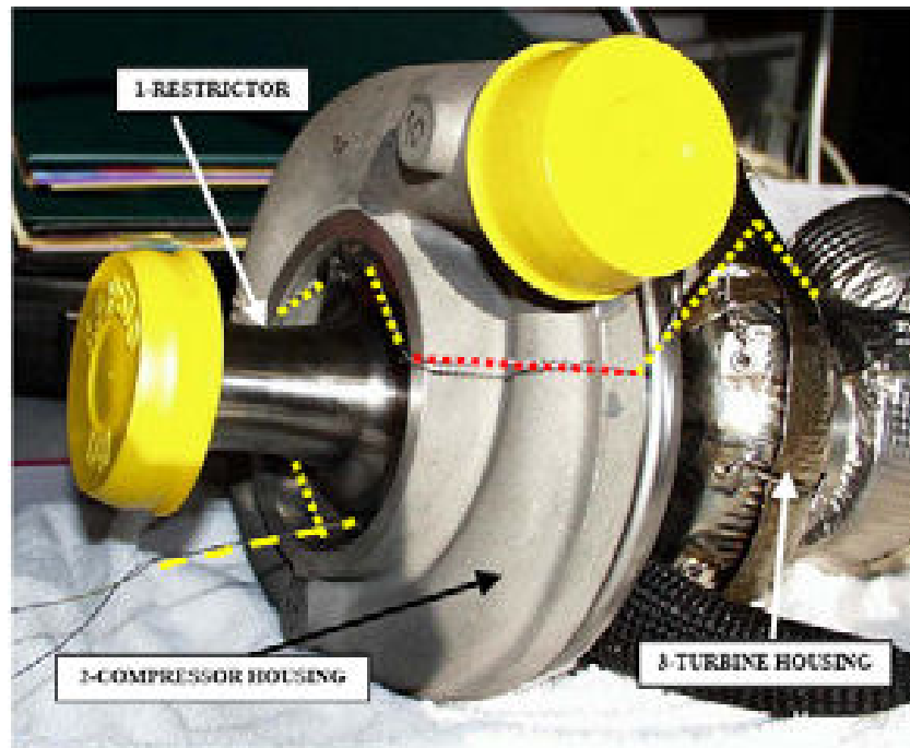
Εικόνα 44: Σφράγιση turbo
