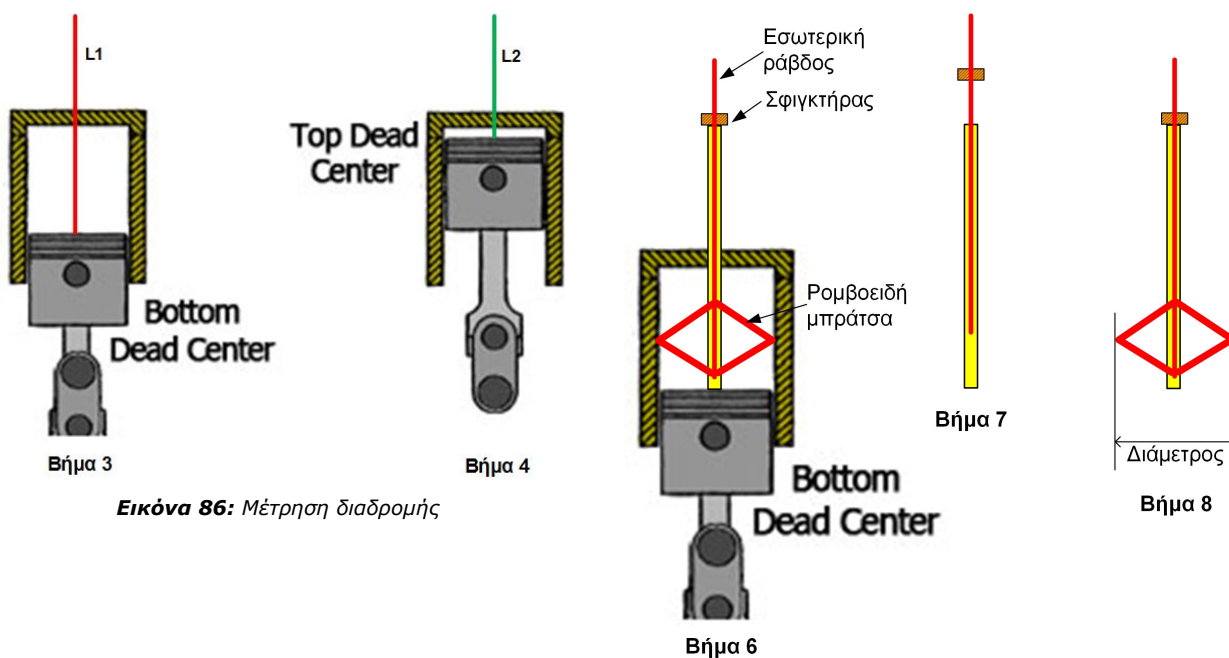
Εικόνα 87: Μέτρηση διαμέτρου
