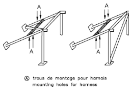
Εικόνα 32: Στήριξη ζωνών ασφαλείας στον κλωβό ασφαλείας
