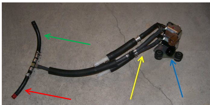
Εικόνα 70: Σωληνάκια ελέγχου waste gate
