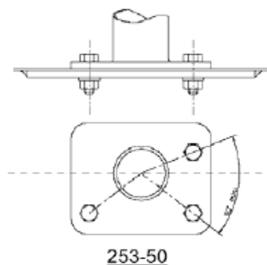
Εικόνα 31: Γωνία βιδών στήριξης κλωβού
