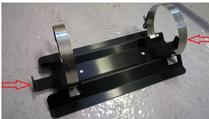
Εικόνα 40: Anti-torpedo tabs
