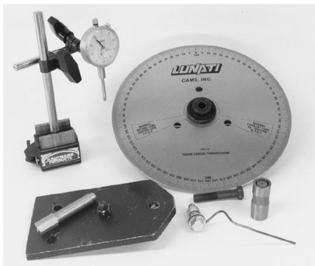
Εικόνα 88: Διάταξη μέτρησης εκκεντροφόρων
